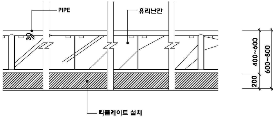
입면
