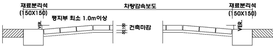
차량감속보도 횡단면도
