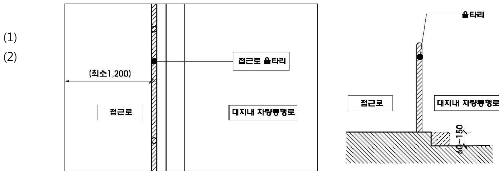
접근로 울타리
