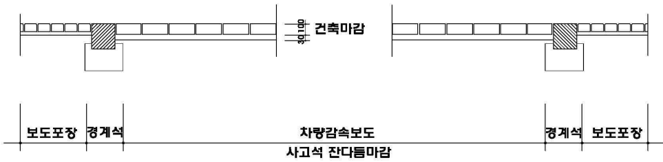
차량감속보도 횡단면도
